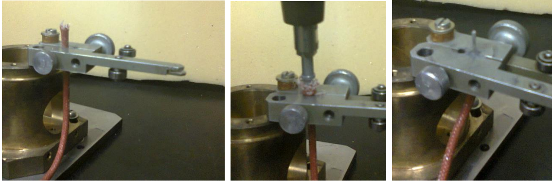
Рисунок 2. Процес зачищення провода
