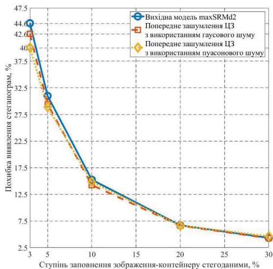
Рисунок 1. Залежність похибки виявлення стеганограм від ступеня заповнення ЗК стегаданними при попередньому зашумленні зображень з використанням адитивного гаусового та пуасонового шумів
